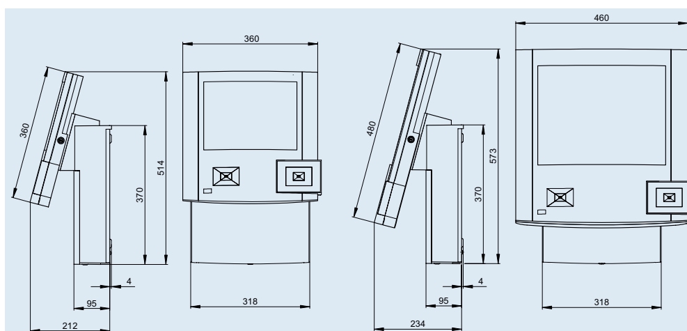
Detaillierte Maßzeichnungen finden Sie als Download auf unserer Homepage. Technische Änderungen vorbehalten! Bestell-Nr. DABL B-Net 95 80, Stand 0906
